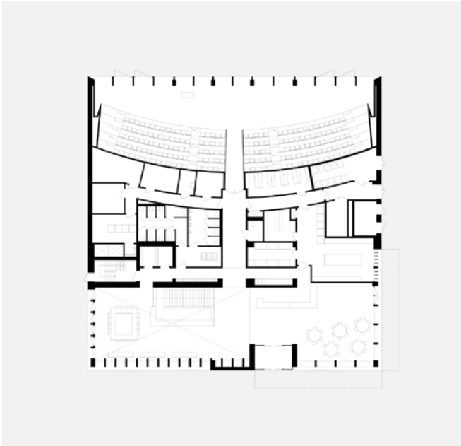
Alle functies, zoals een café zijn zorgvuldig geplaatst in de ruimte tussen de grote foyer en de hoofdcollegezaal.
