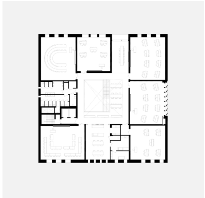
Op de bovenste verdieping is er meer ruimte gewijd aan individuele studie.
